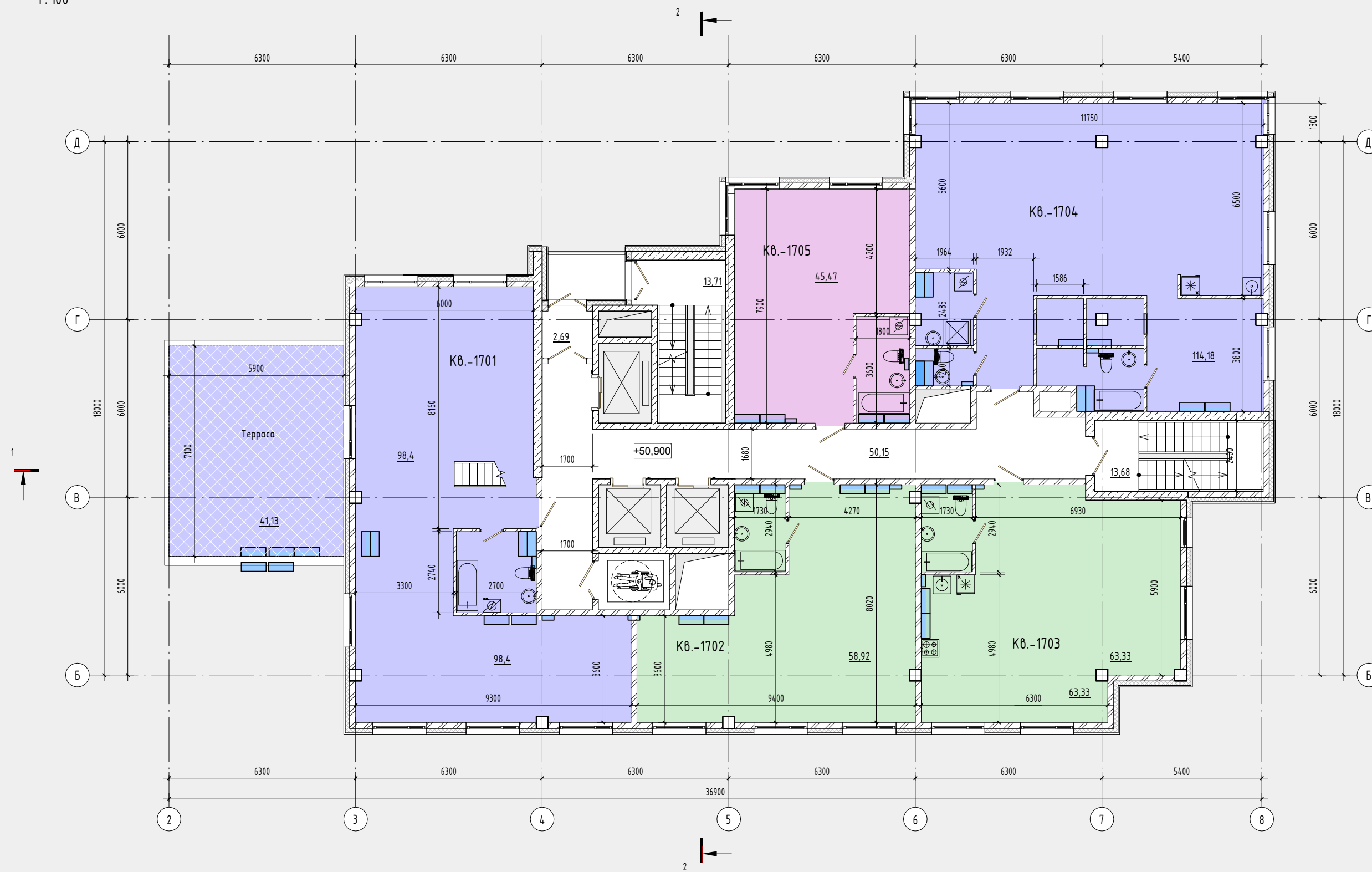
Экспликация помещений + 17 Этаж
