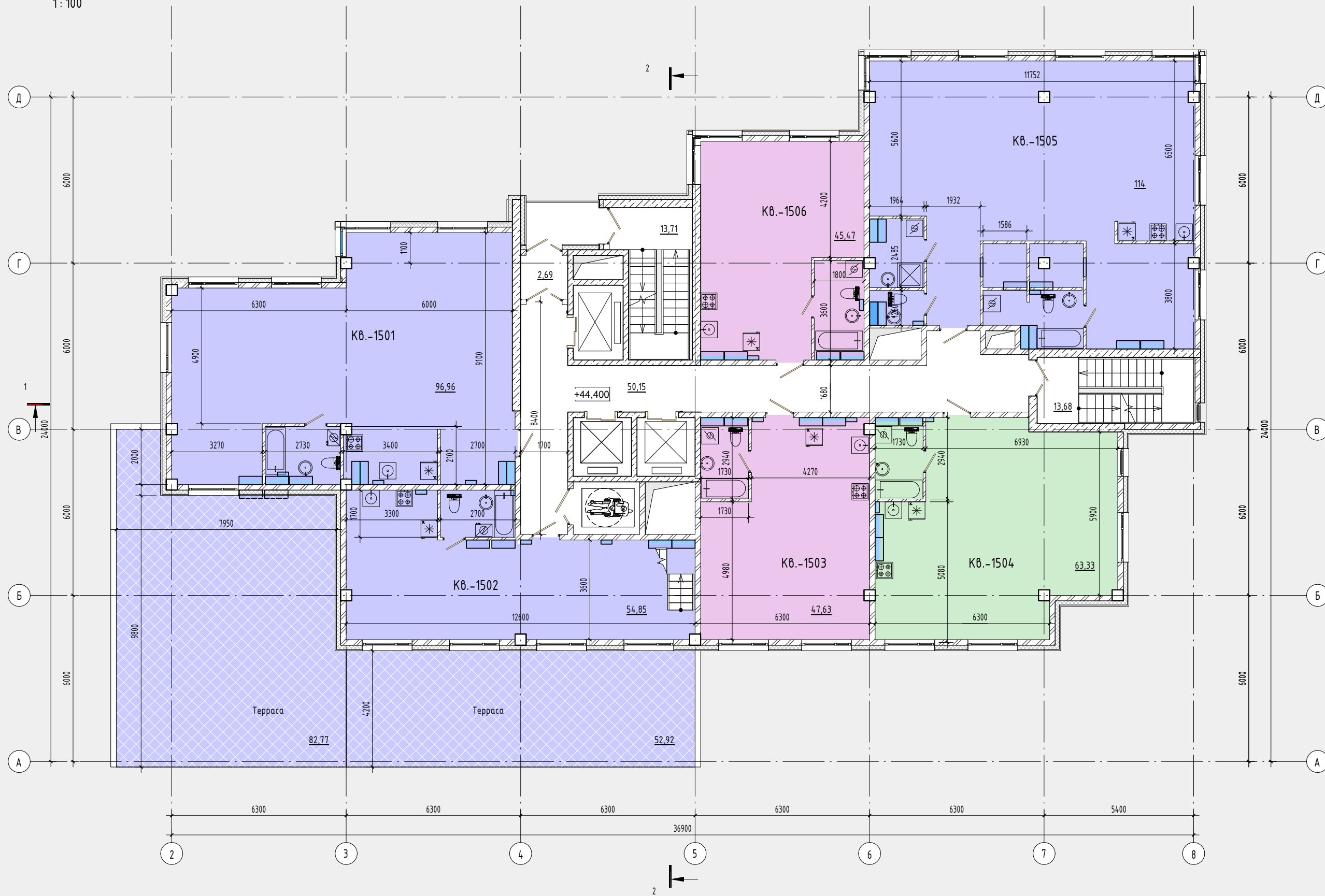
Экспликация помещений + 15 Этаж
